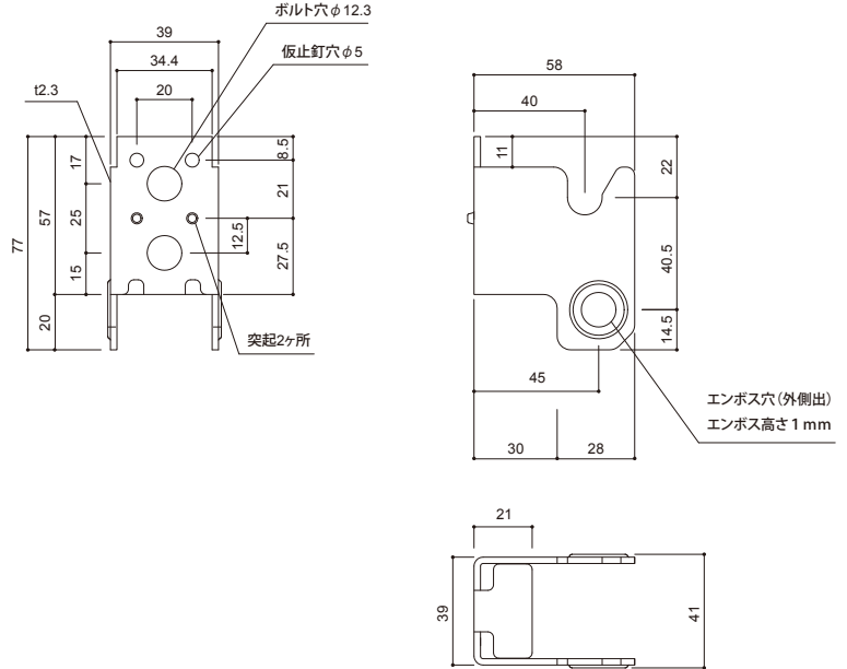
■仕様図
