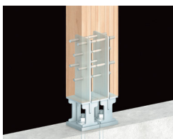
複数使いが可能な高耐力の柱脚金物「MP柱脚システム」
