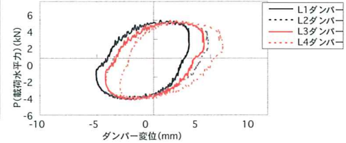
ダンパー変位グラフ(D1試験体、1/30rad)
