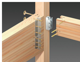
金物工法(大梁・燃えしろ対応) 「プレセッターSU」
