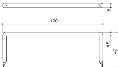
■仕様図
