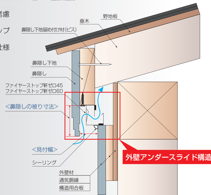
<図1> 施工断面図
