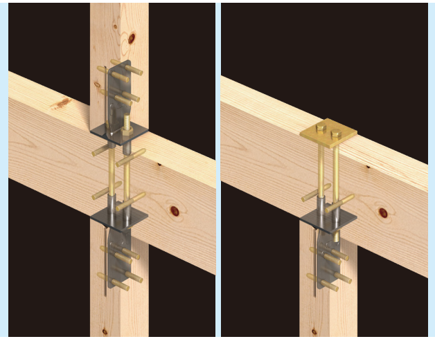
両引きセット使用例
