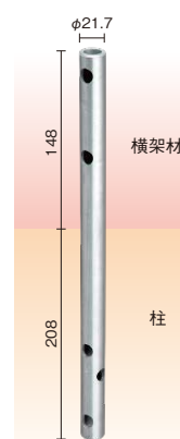
PZ-HDP-20CN ※横架材の梁成が180mmの場合
