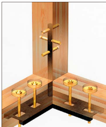
●コーナータイプ PSHD-30CN-II(105用) PSHD-30CN(120用)
